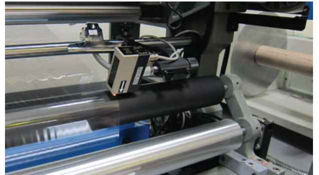
Renk Çizgi Sensör DLP-09 kenar pozisyon kontrol üzerinde kullanılmaktadır.
